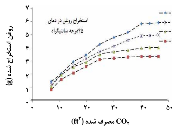
شکل ۴- استخراج روغن به وسیله \text{CO}_2 فوق بحرانی از 19.8 گرم روغن کارکرده در دمای 45 درجه سانتیگراد و فشارهای گوناگون.
