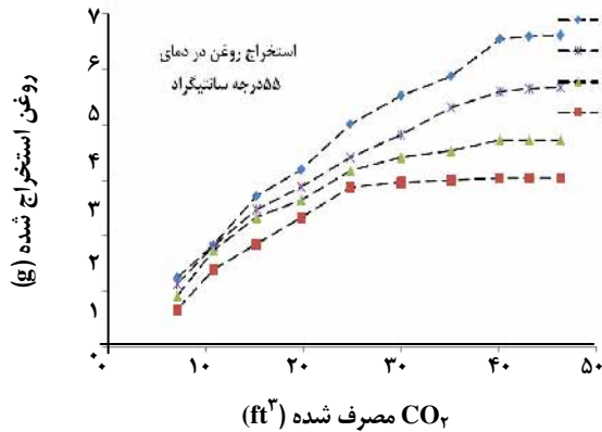
شکل ۵- استخراج روغن به وسیله \text{CO}_2 فوق بحرانی از 19.8 گرم روغن کارکرده در دمای 55 درجه سانتیگراد و فشارهای گوناگون.
