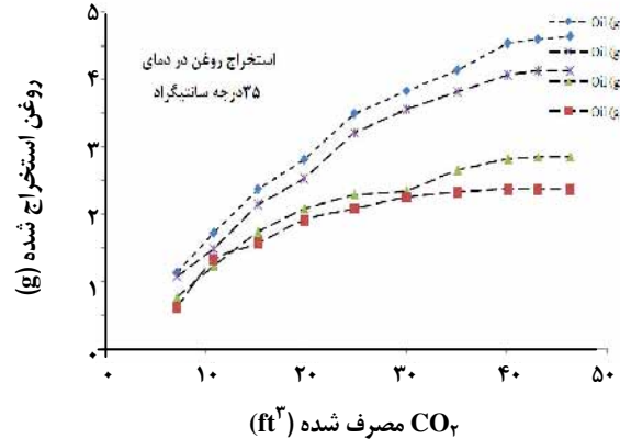
شکل ۳- استخراج روغن به وسیله \text{CO}_2 فوق بحرانی از 19.8 گرم روغن کارکرده در دمای 35 درجه سانتیگراد و فشارهای گوناگون.
