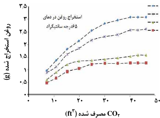
شکل ۶- استخراج روغن به وسیله \text{CO}_2 فوق بحرانی از 19.8 گرم روغن کارکرده در دمای 65 درجه سانتیگراد و فشارهای گوناگون.
